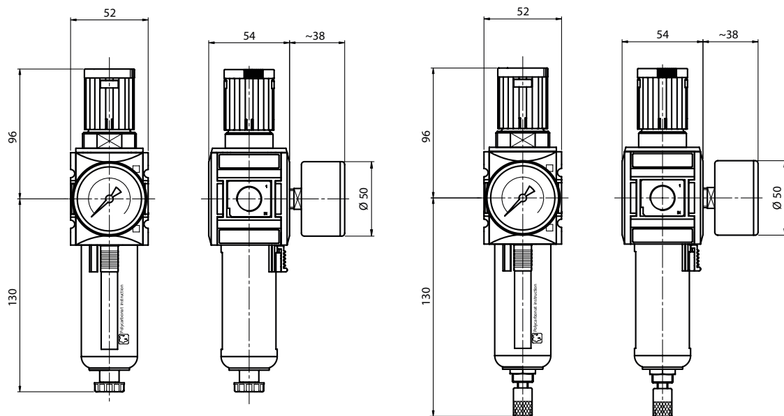
félautomata leeresztés
