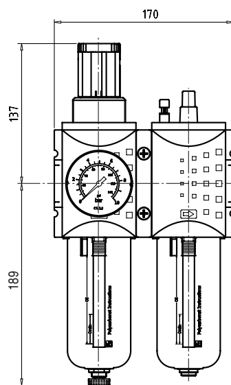
félautomata leeresztés
