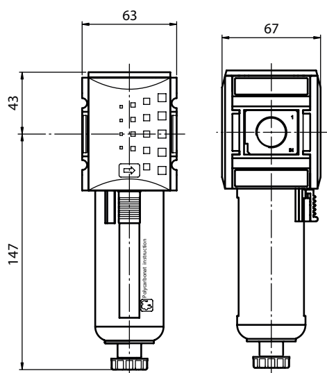
félautomata leeresztés
