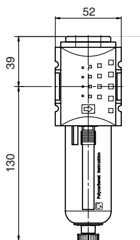
félautomata leeresztés
