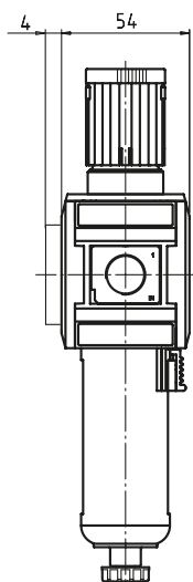
félautomata leeresztés
