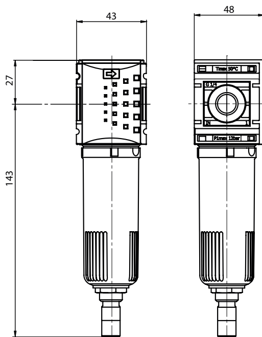
automata leeresztés
