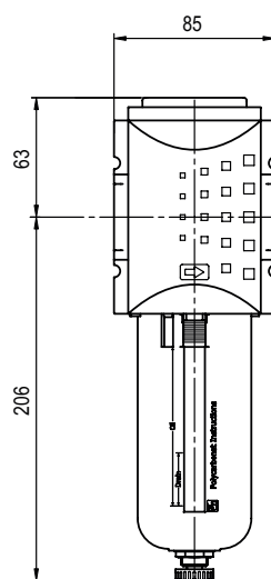
automata leeresztés
