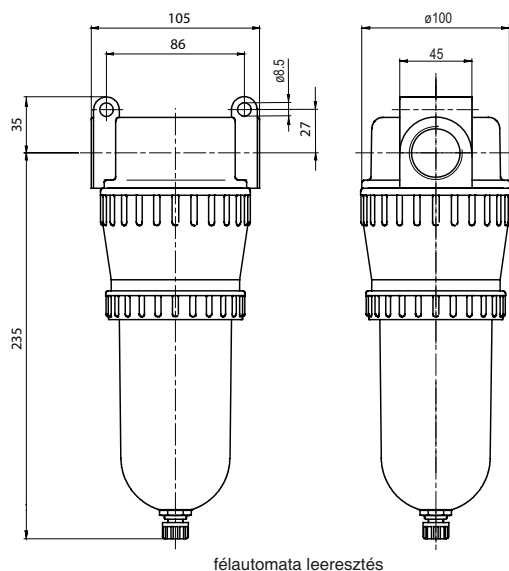
félautomata leeresztés
