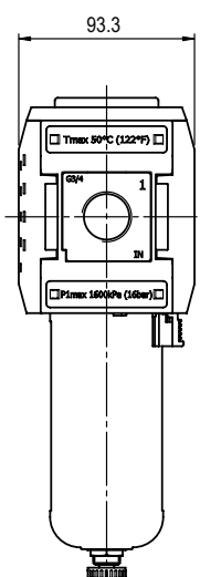
félautomata leeresztés
