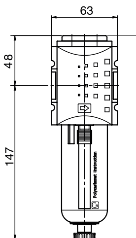
félautomata leeresztés
