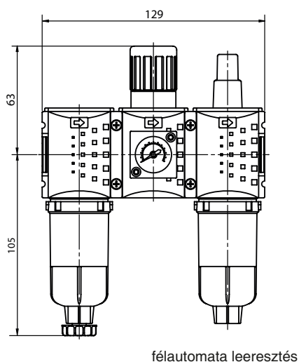
félautomata leeresztés
