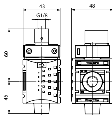
pneumatikus vezérlésű
