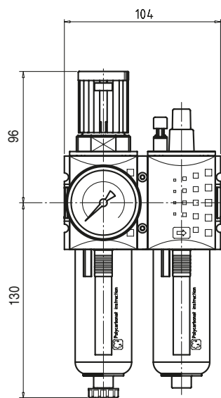
félautomata leeresztés
