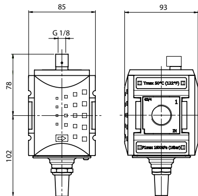
pneumatikus vezérlésű
